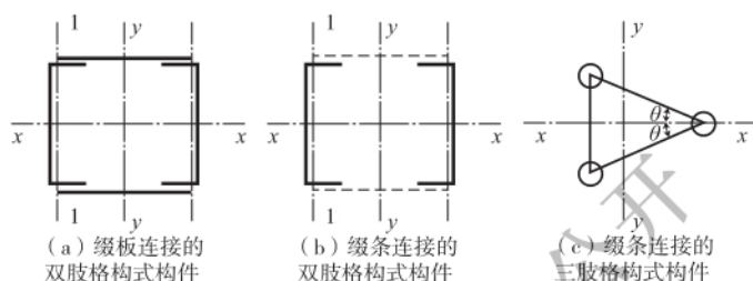
图 5.2.6 格构式构件截面示意图
