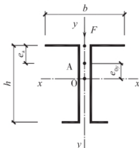
图 B. 2. 2 单轴对称截面示意图
