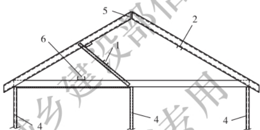
(b) 斜梁
