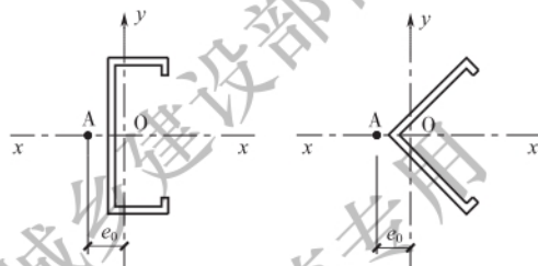
图 5.2.4 单轴对称开口截面示意图
