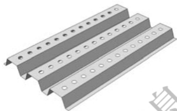
图 8.1.10 压型钢板翼缘开圆孔示意图
